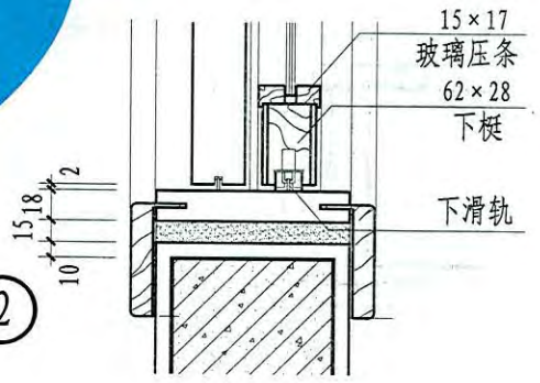
F型-推拉窗节点图 (一)
