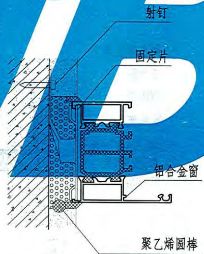
③ 钢筋混凝土墙体
