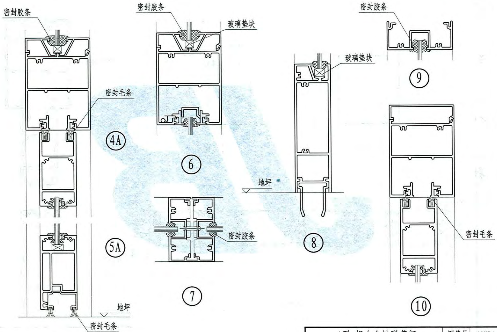
A型-铝合金地弹簧门 基本门节点图(二)
