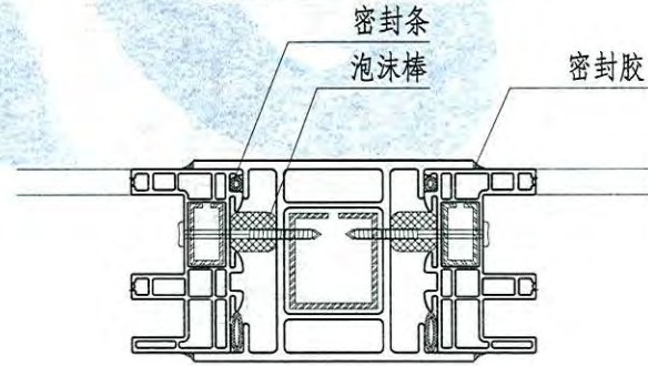
D型—塑料组合门窗拼接节点图
