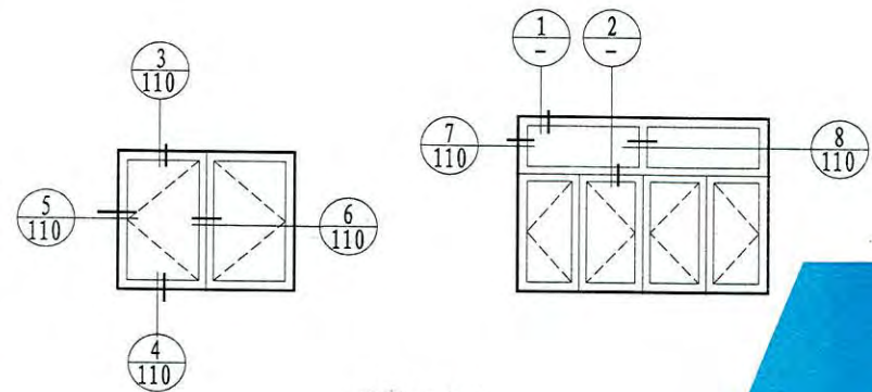
窗立面图
