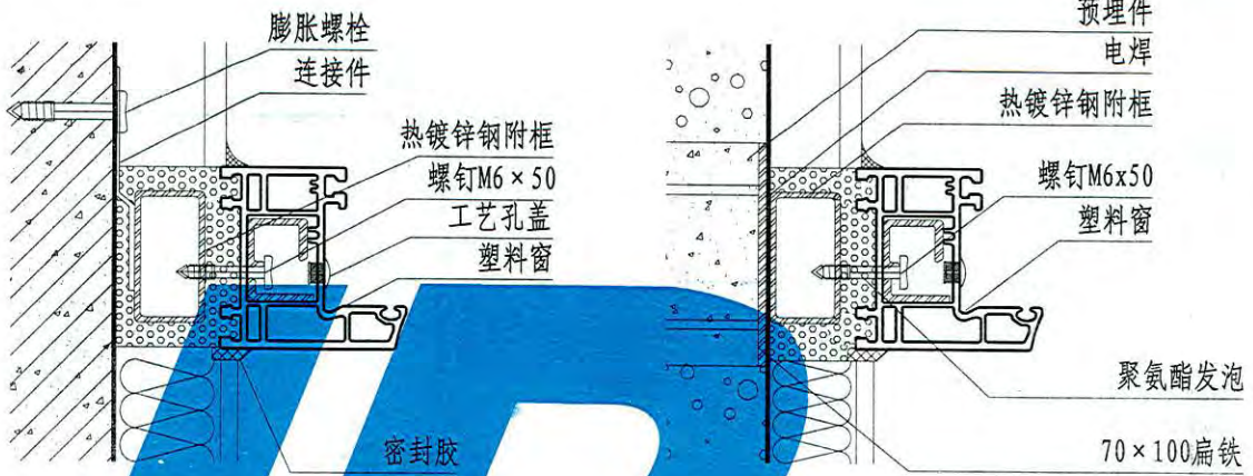
① 混凝土附框安装
