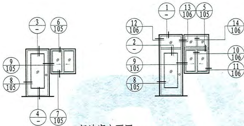
门连窗立面图
