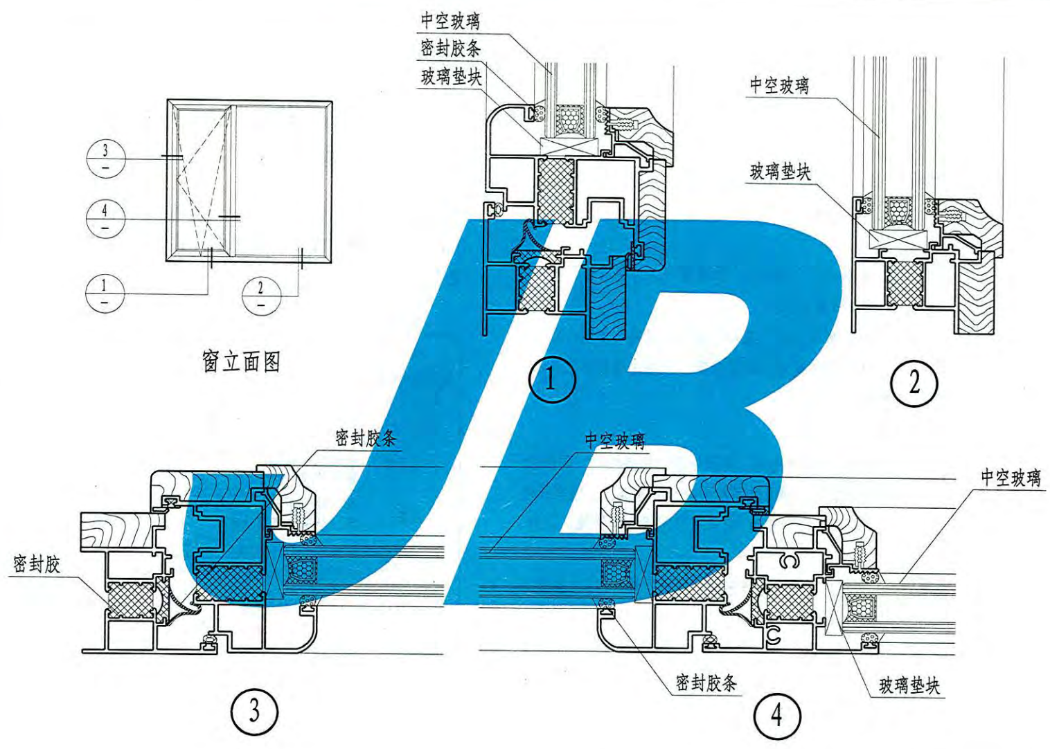
C型-木包铝平开下悬窗节点图 图集号 12YJ4-1 页次 53
