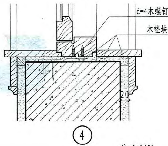
平开门连窗安装节点图
