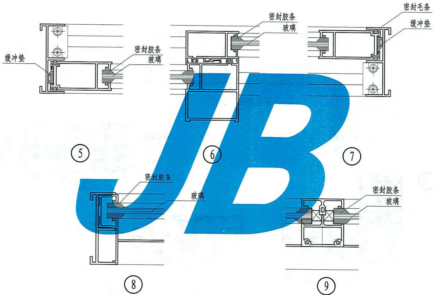
A型-铝合金推拉 单玻门节点图(二) 图集号 12YJ4-1 页次 33
