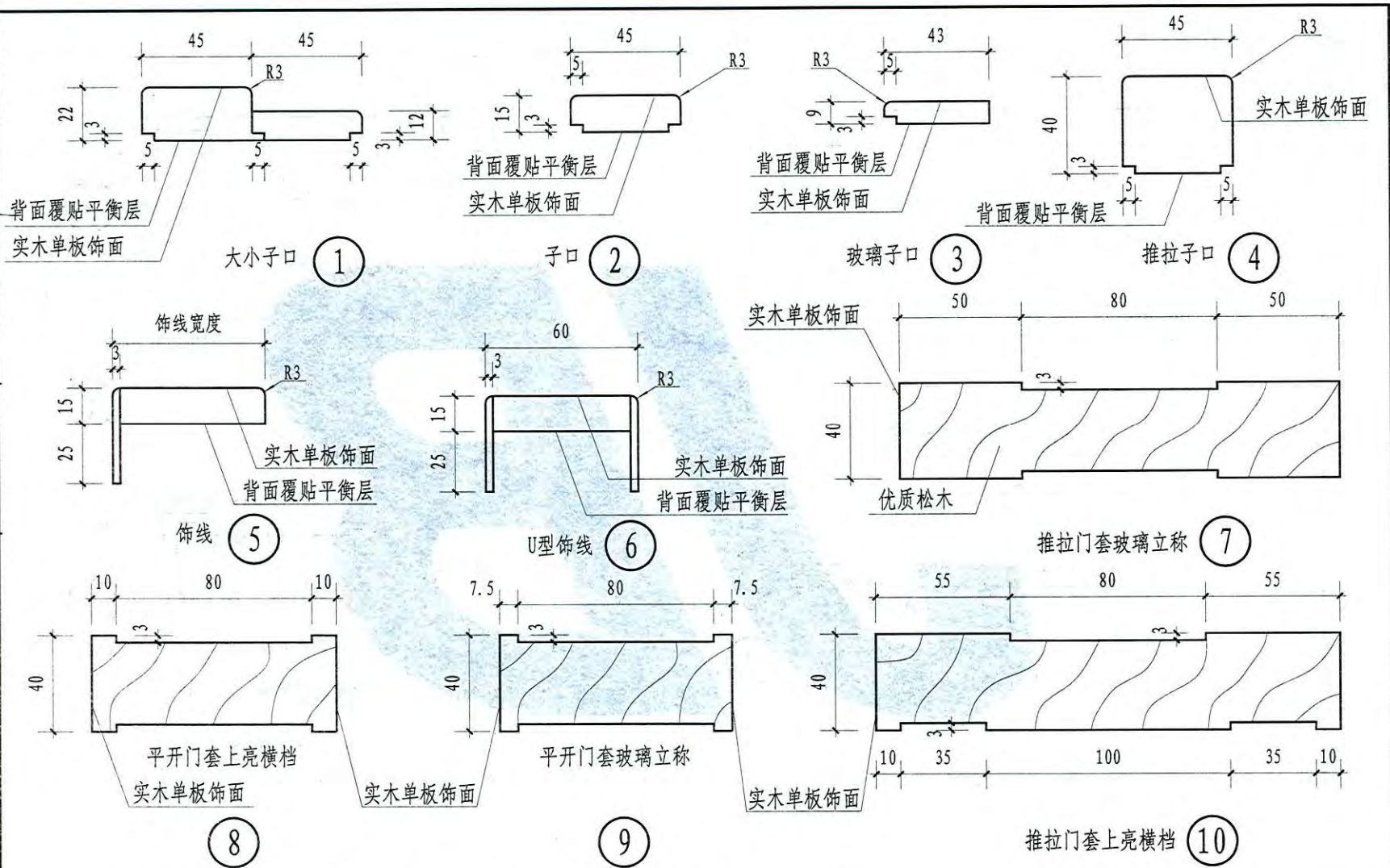
门窗套部件截面图(二)
