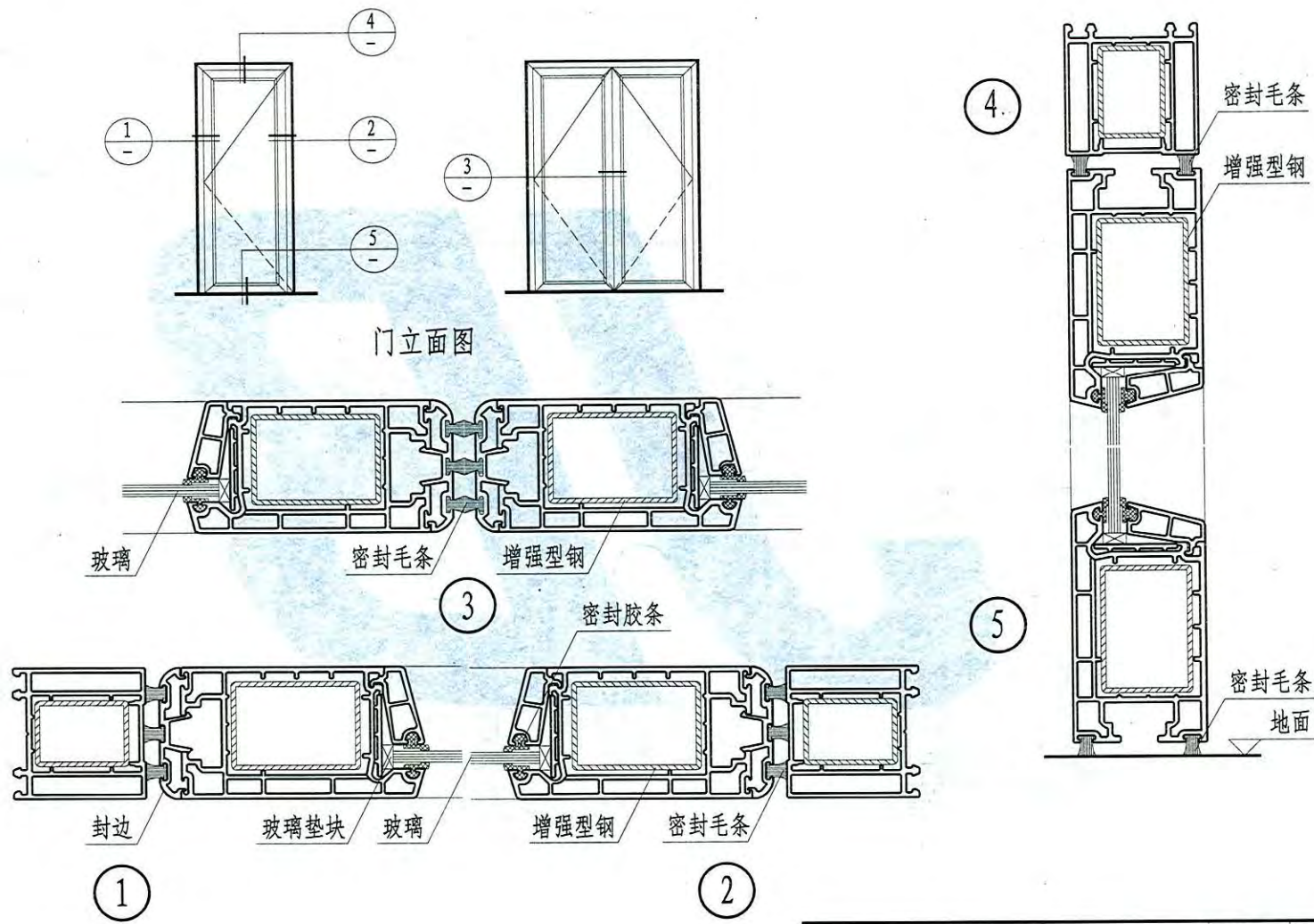
D型—塑料地弹簧门节点图
