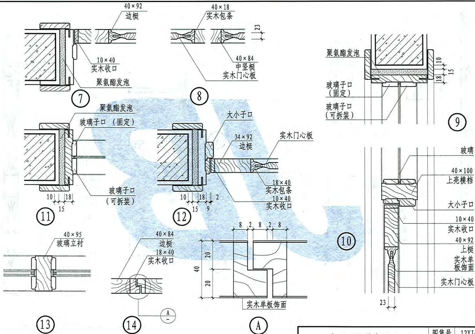
F型-平开门节点图 (二)
