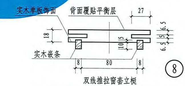
门窗套部件截面图 (一) 图集号 12YJ4-1 页次 113
