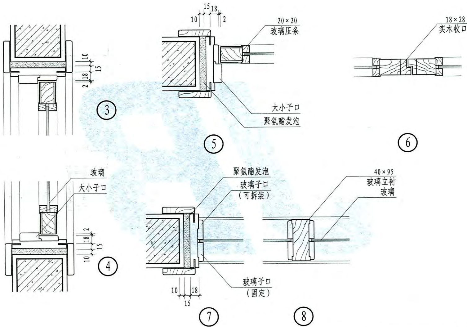
F型-室内平开窗节点图(二)
