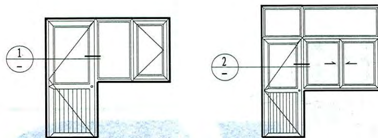
门连窗立面图
