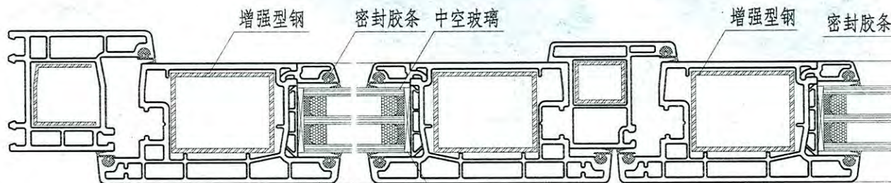
D型—塑料外平开门节点图 (带门芯板)
