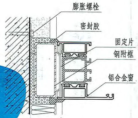
① 附框安装
