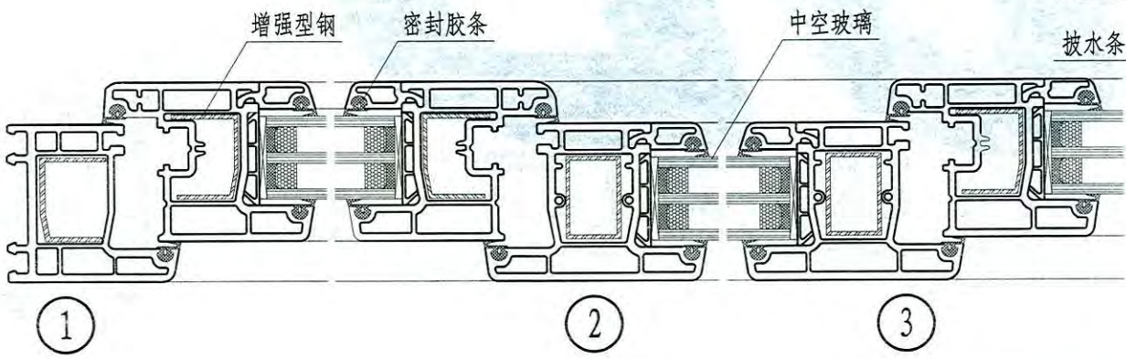
D型—塑料内平开下悬窗节点图
