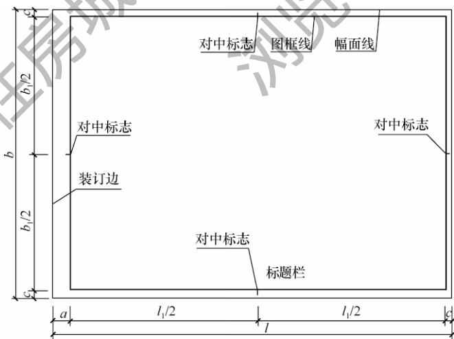
图 3.2.1-2 A0~A3 横式幅面 (二)
