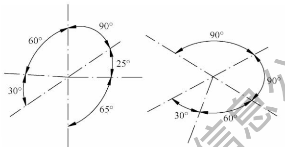
图 10.5.6 轴测图角度的标注方法
