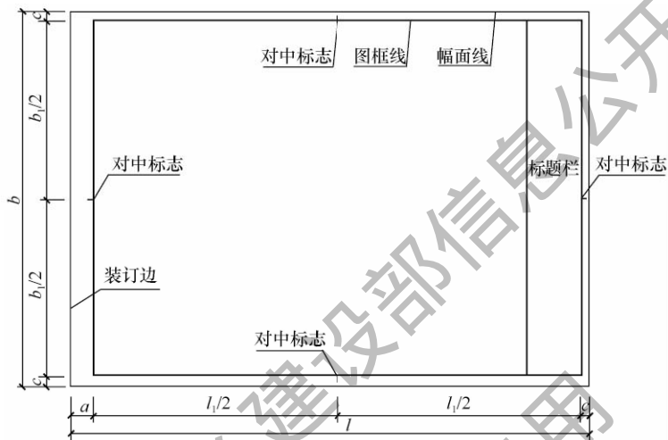
图 3.2.1-1 A0~A3 横式幅面 (一)
