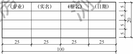
图 3.2.2-5 会签栏
