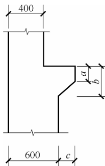
图 11.7.6 相似构配件尺寸表格式标注方法
