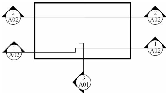
图 7.1.3 剖视的剖切符号（一）
