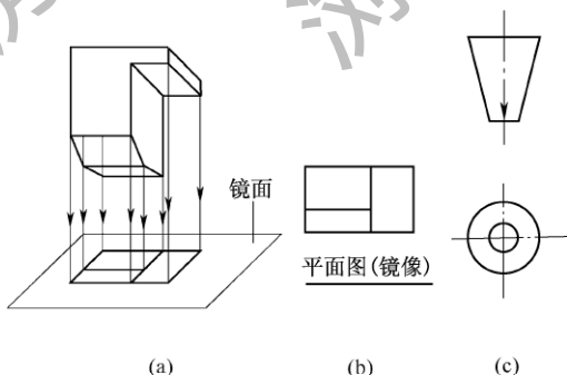
图 10.1.2 镜像投影法
