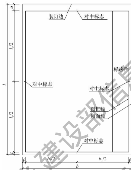
图 3.2.1-5 A0~A4 立式幅面 (二)
