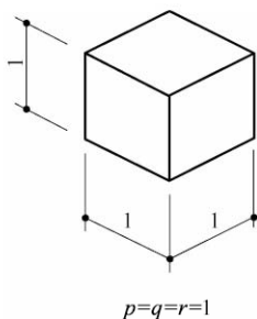
图 10.5.1 正等测的画法
