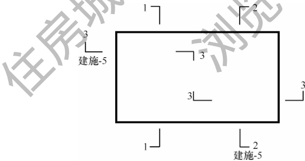
图 7.1.4-1 剖视的剖切符号（二）
