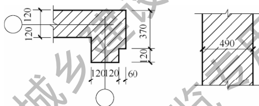
图 11.3.1 尺寸数字的注写
