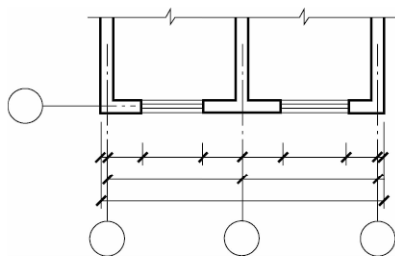
图 11.3.2 尺寸的排列
