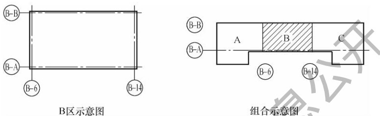
图 10.2.3 分区绘制建筑平面图
