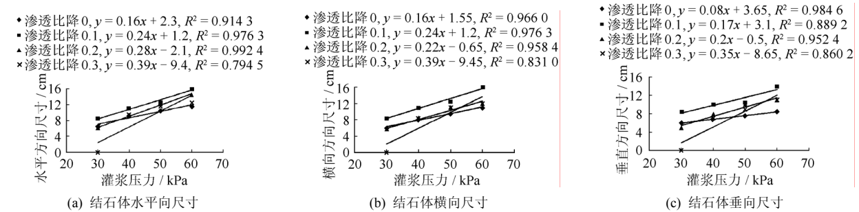
图 7 不同渗透比降条件下有渗流作用结石体尺寸随灌浆压力变化情况
