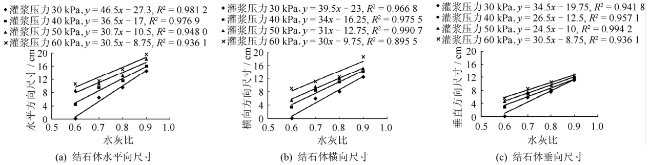
图 6 不同灌浆压力条件下无渗流作用结石体尺寸随水灰比变化情况
