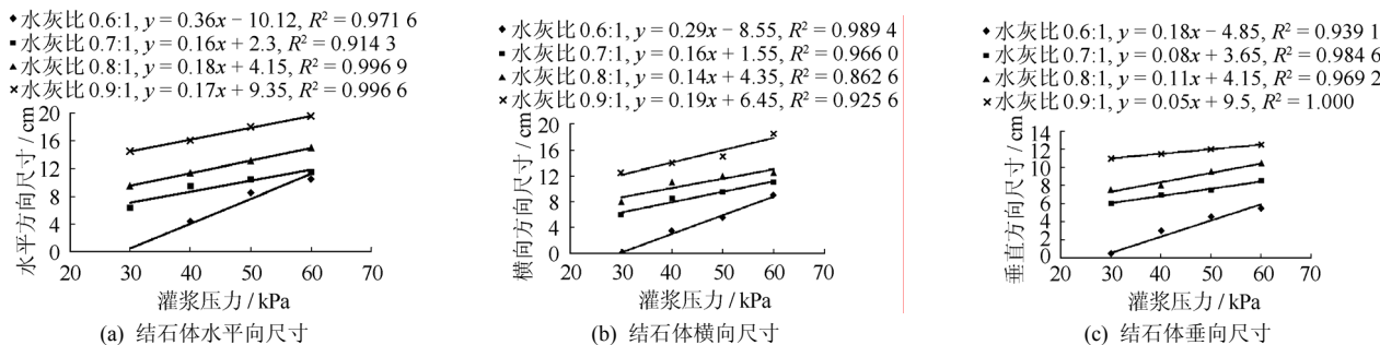
图 5 不同水灰比条件下无渗流作用结石体尺寸随灌浆压力变化情况
